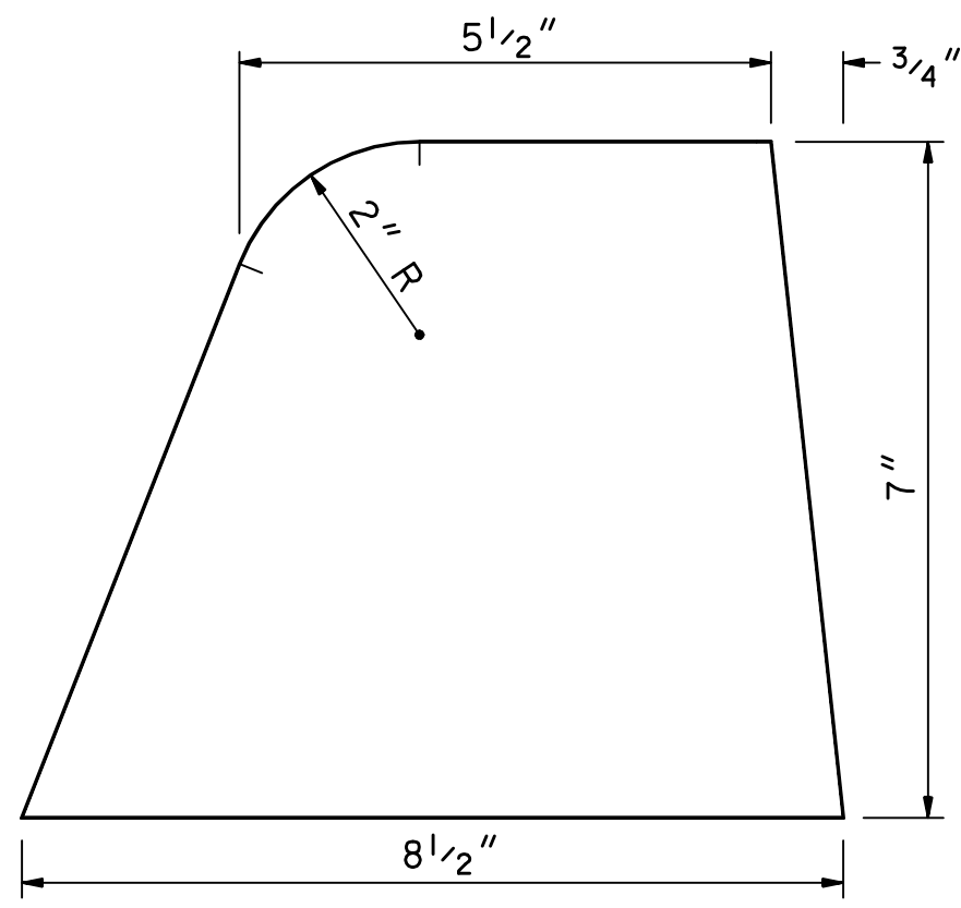
TYPE 'A' ITEM 609.812
